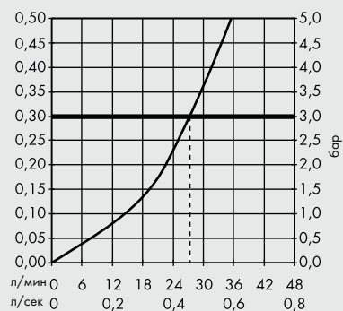
Расходные характеристики при свободном истечении.
