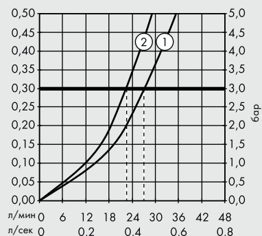
Расходные характеристики при свободном истечении.
