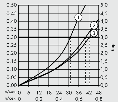
Расходные характеристики при свободном истечении.
