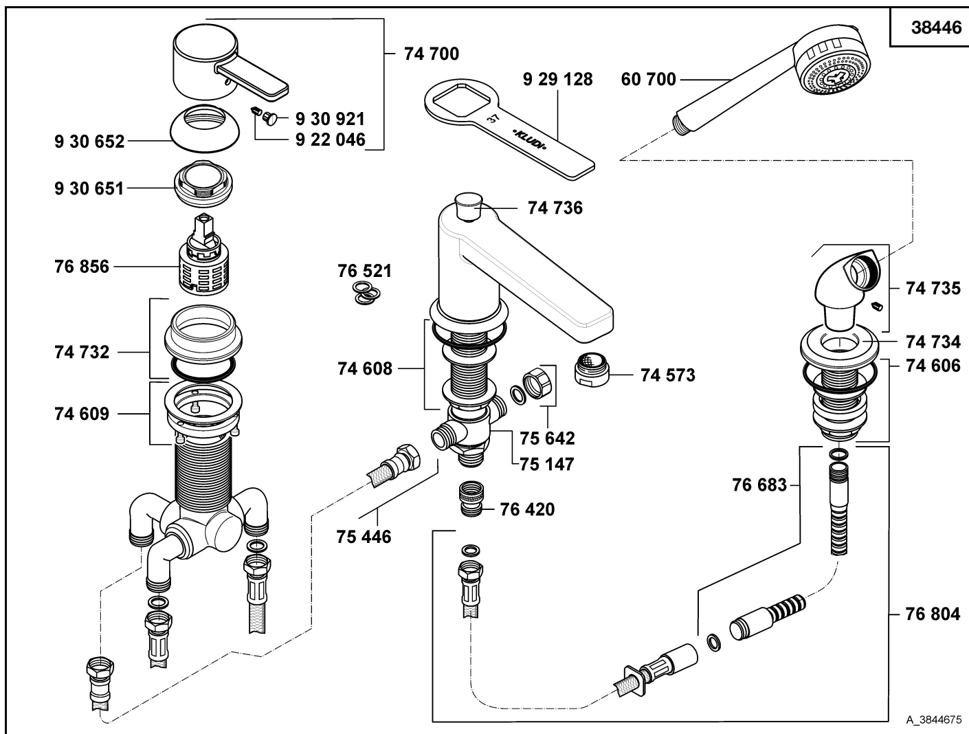
38446 Wannenfüll- und Brause- Einhandmischer DN 15 single lever bath- and shower mixer DN 15 ééngreeps bad-/douchemengkraan 1/2"
