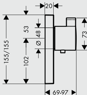
ShowerSelect® Thermostat Highflow für 1 Verbraucher (unten) und einen zusätzlichen Verbraucher (oben) # 15761, -000
